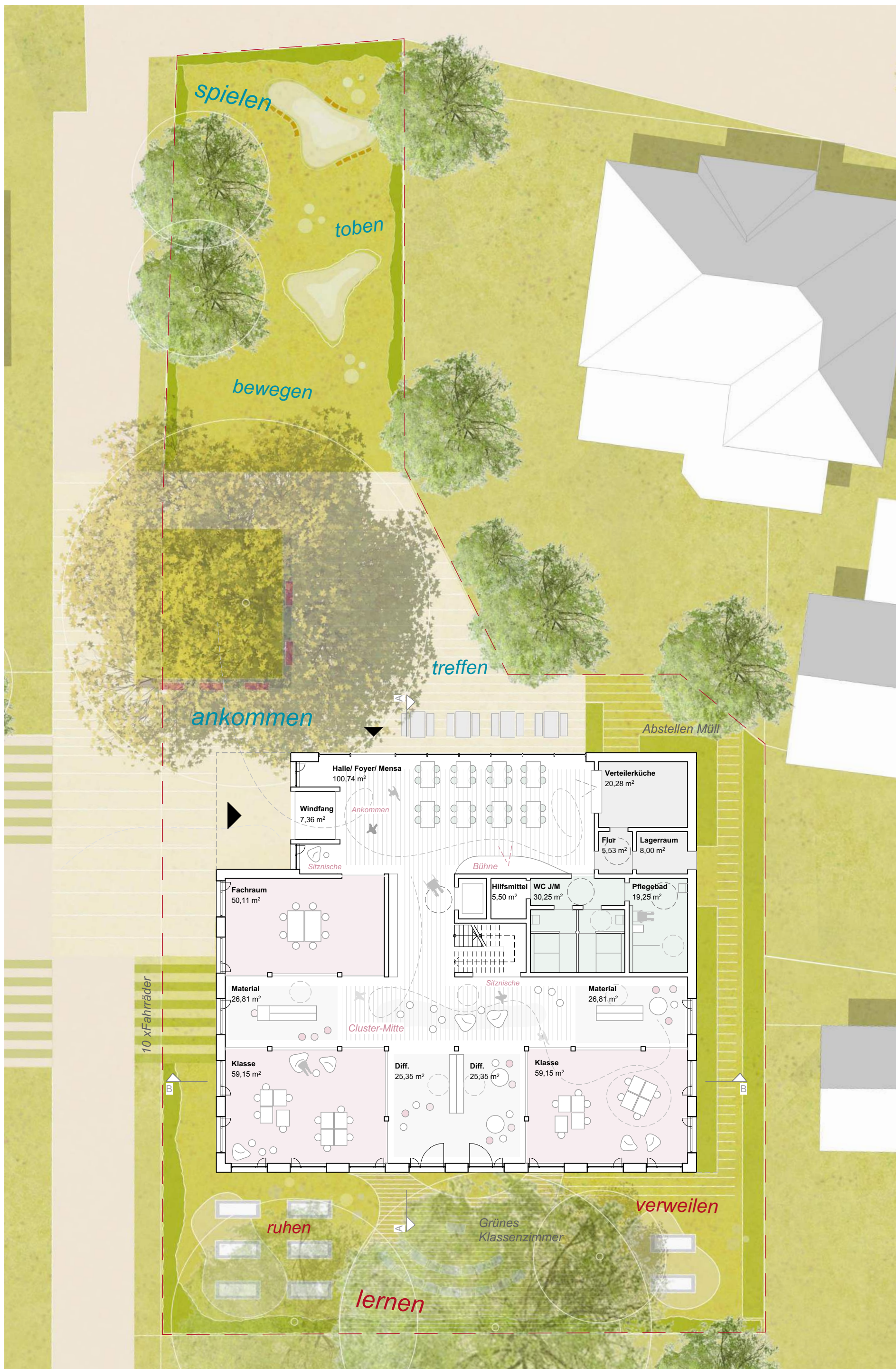
Ergeschoss M 1|200
