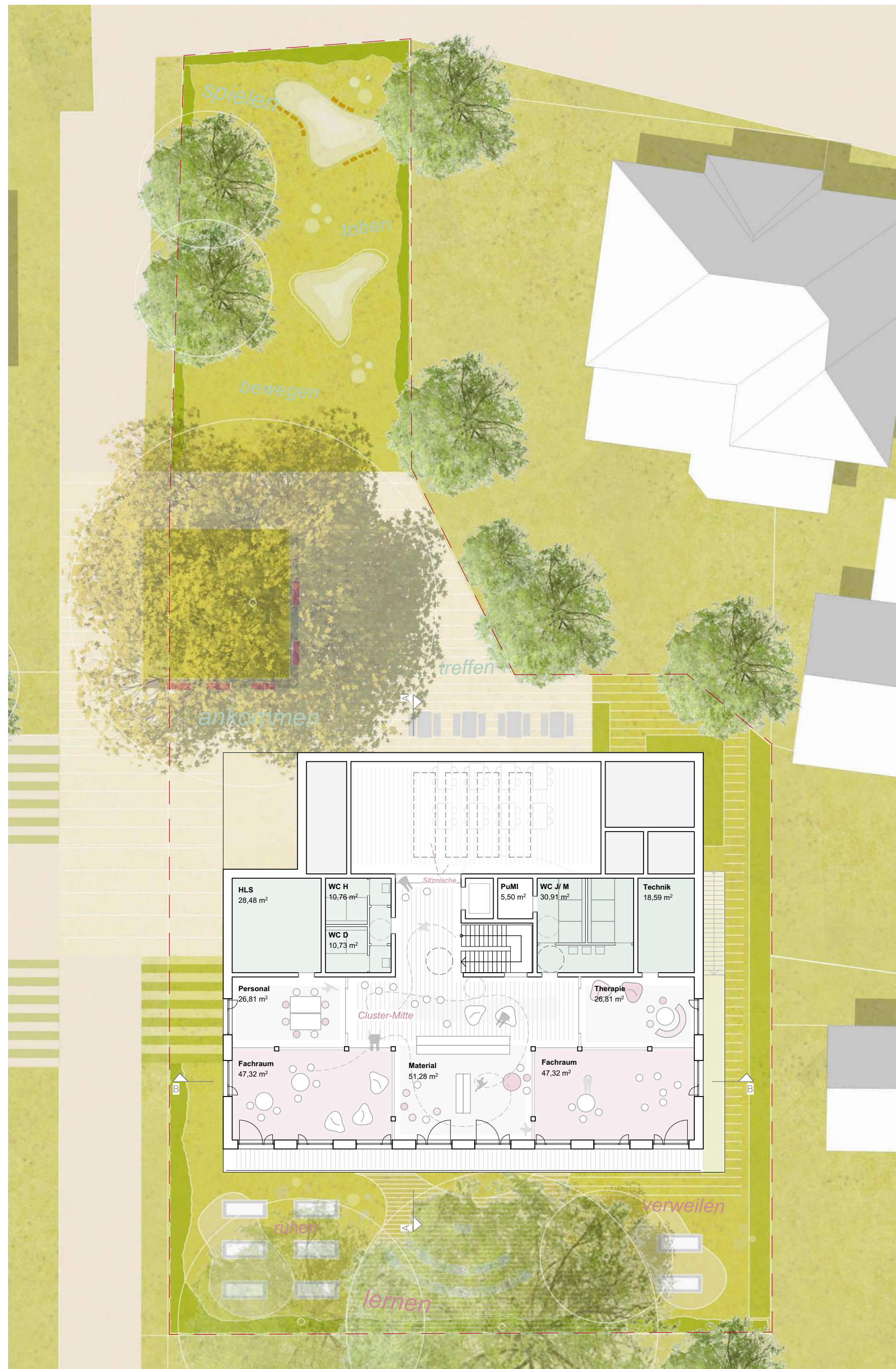
Obergeschoss M 1|200
