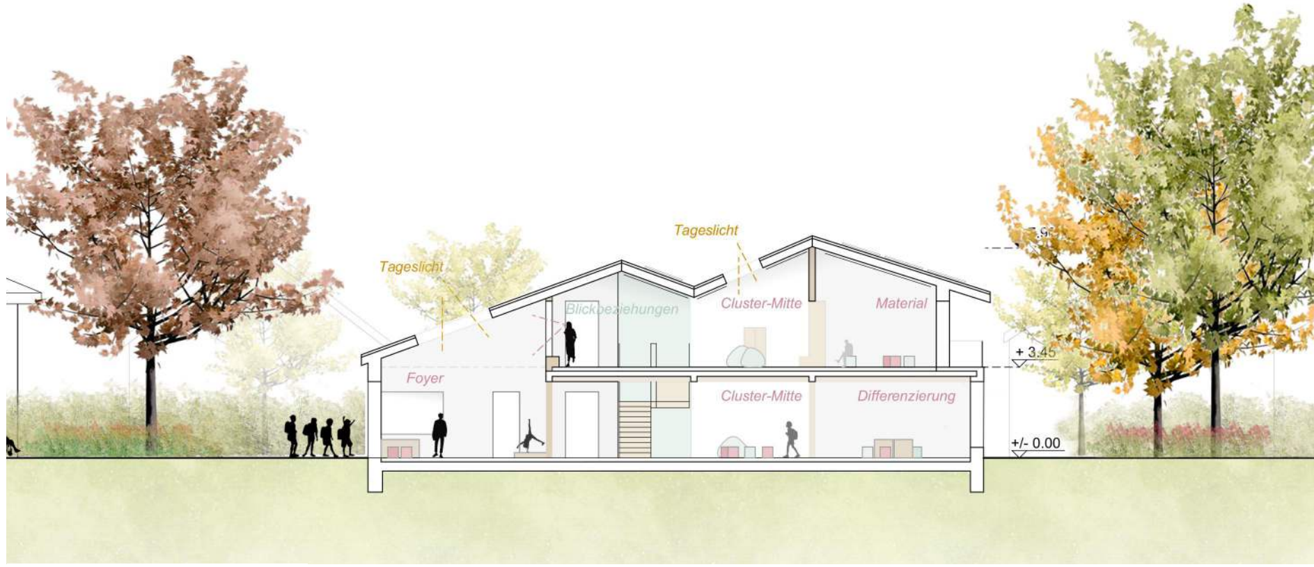
Schnitt A M 1|200
